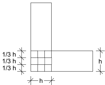
Aufsicht M1:5
