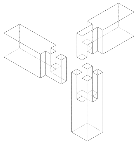
Isometrie
