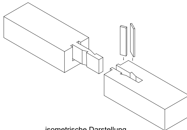
isometrische Darstellung
